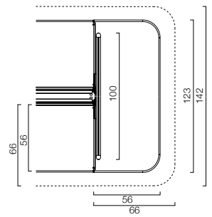
testata con telaio asolato head with slotted frame
