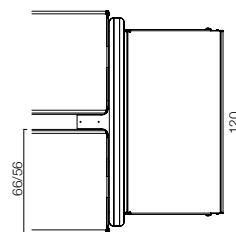
testata con cornice head with frame
